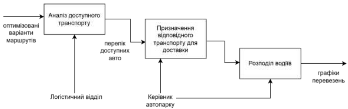
Рисунок 20 - Декомпозиція підпроцесу Призначення транспорту та водіїв
