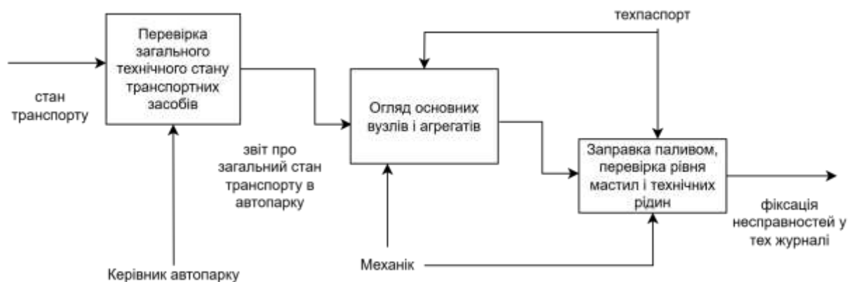
Рисунок 30 - Декомпозиція підпроцесу Щоденний технічний контроль автопарку
