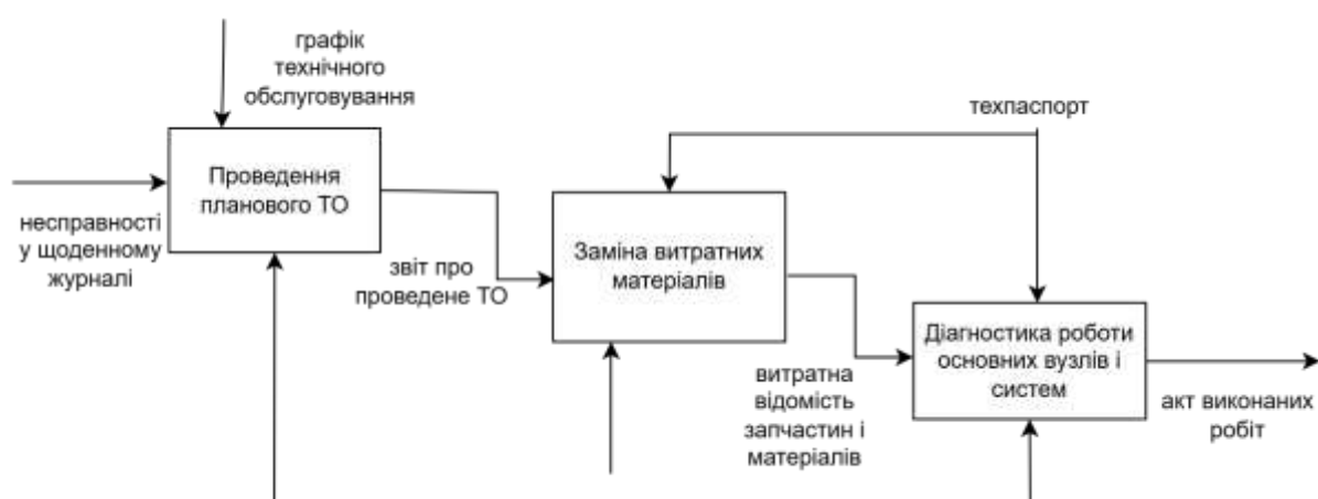
Рисунок 31 - Декомпозиція підпроцесу Регулярне технічне обслуговування
